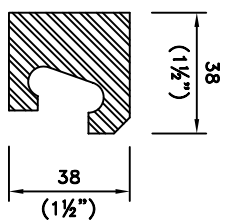
PERFIL DE ACERO PARA "E" GUARDACANTOS" TIPO "E"
